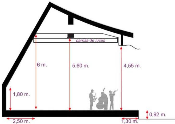
///Sección escenario
