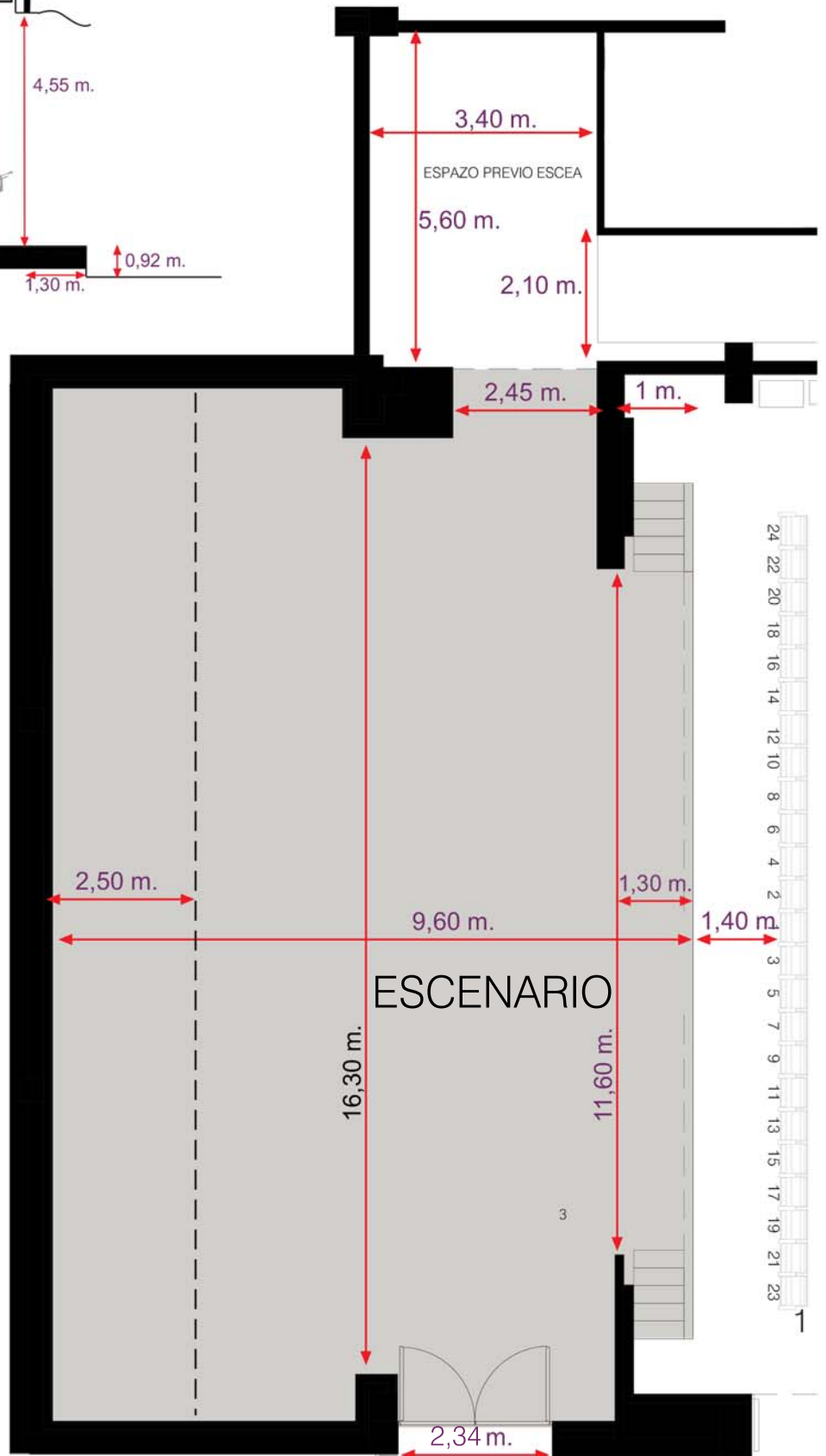
///Planta escenario
